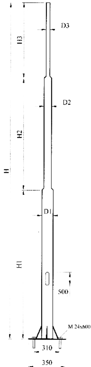
Troetažni cevasti stub sa anker pločom tipa URA
